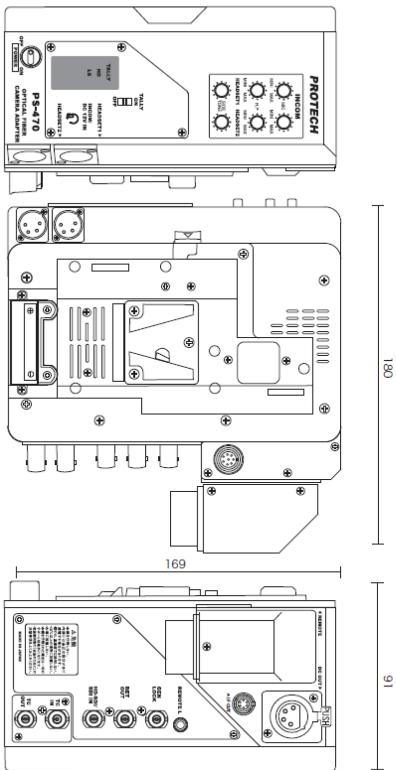
Outside dimension (unit: mm) 外形寸法図(単位:ミリ)
